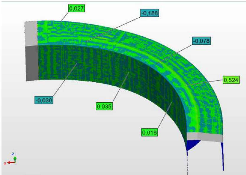
CAD morphed deviations
